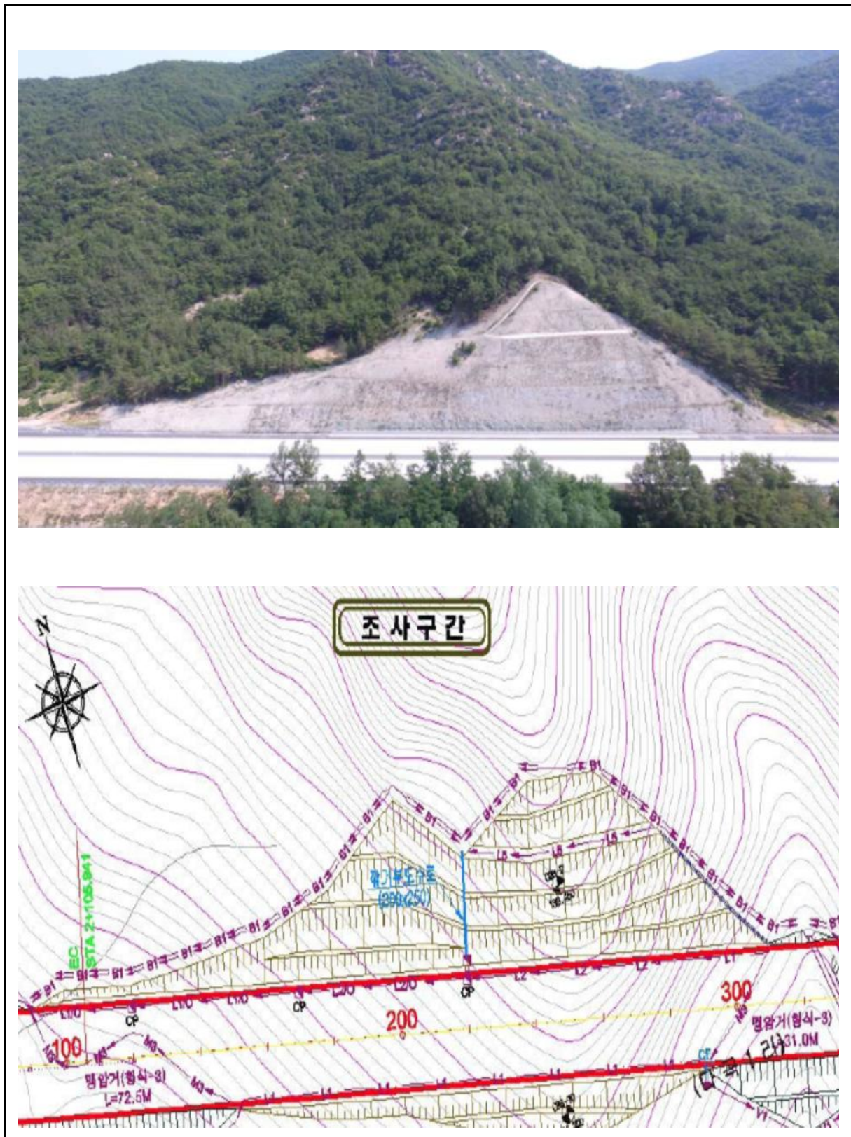
【그림 15.14】 부산·울산선 검토대상 비탈면구간
